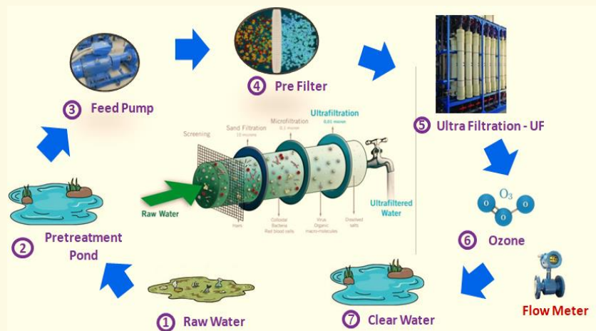
กระบวนการบำบัดน้ำด้วยระบบอัลตราฟิลเตรชัน (Ultrafiltration) และกำจัดเชื้อด้วยระบบโอโซน (Ozone)
