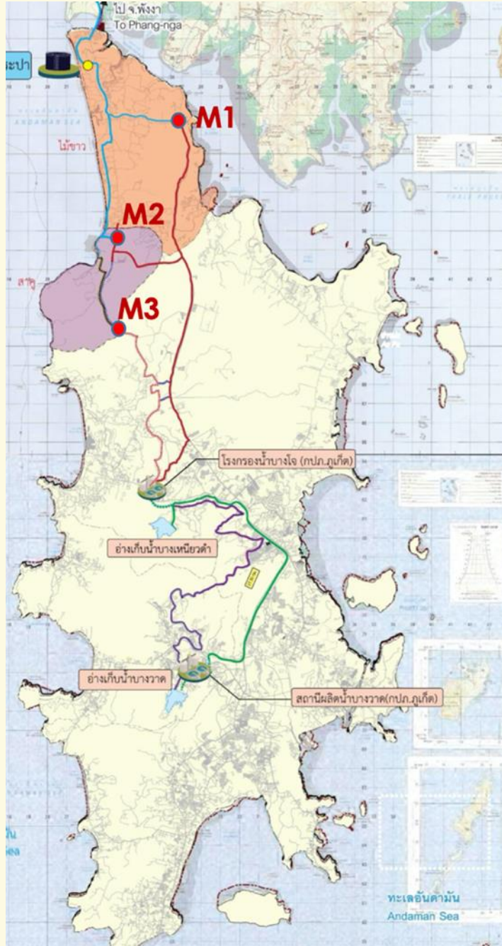
รูปภาพแนวการต่อเชื่อมต่อของ GS กับแนวท่อของ กปภ.
